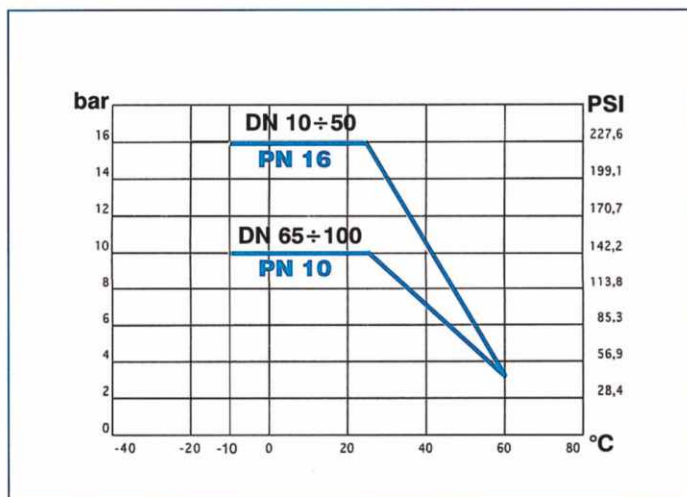
GRÁFICO PRESIÓN - TEMPERATURA
