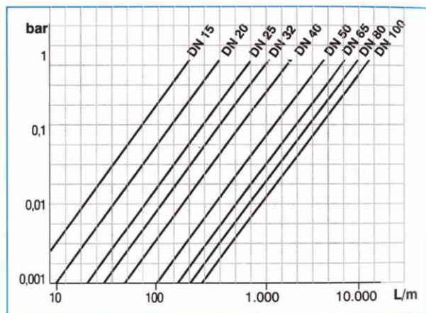
GRÁFICO PERDIDAS DE CARGA
